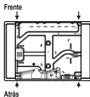
Posição do gancho para H=30mm
