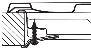
Posición del gancho para superficies H=40\text{mm}
