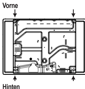
Position der Haken für Arbeitsplatten H=30mm
