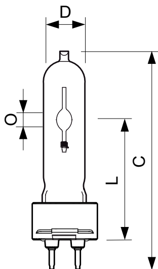
CDM-T Evolution 35 W /930
