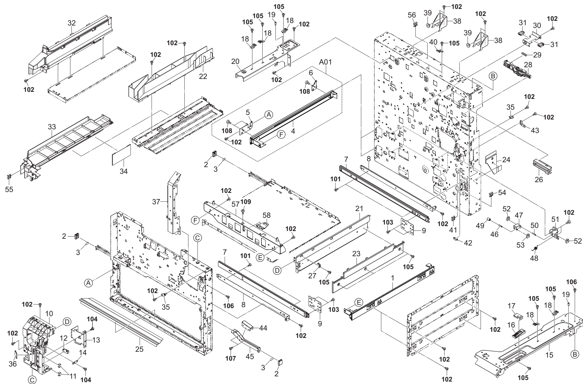
FIG. 4 Frames
