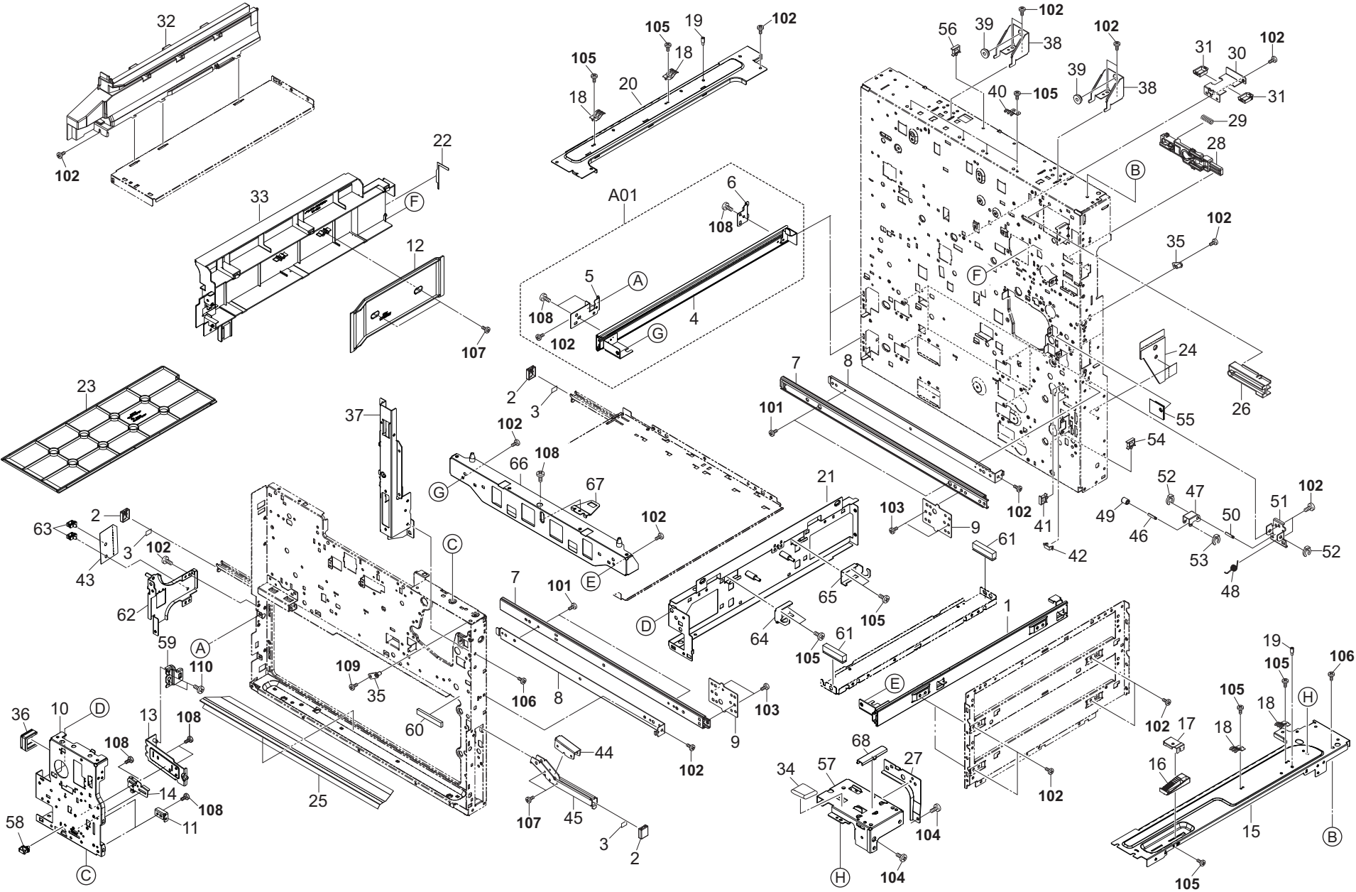
FIG. 4 Frames
