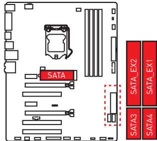
1xM.2 SATA SSD + 2xSATAe HDDs + 2xSATA HDDs
