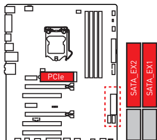
1xM.2 PCIe SSD + 2xSATAe HDDs
