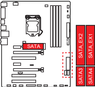
1xM.2 SATA SSD + 2xSATAe HDDs + 2xSATA HDDs
