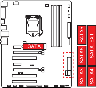
1xM.2 SATA SSD + 1xSATAe HDD + 4xSATA HDDs
