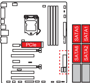
1xM.2 PCIe SSD + 4xSATA HDDs
