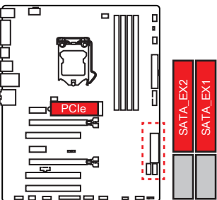
1xM.2 PCIe SSD + 2xSATAe HDDs
