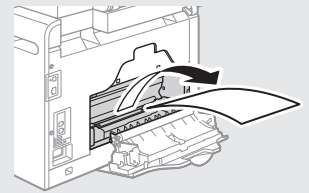
الجانب الخلفي
