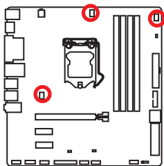
Lüfteranschluss des Spannung-Modus
