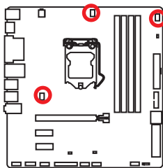
Разъем вентилятора режима напряжения
