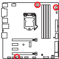
Connecteurs pour ventilateurs en mode tension
