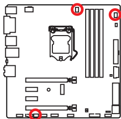
Разъем вентилятора режима напряжения
