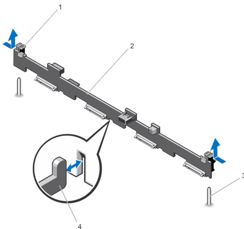
Figure 47. Retrait et installation du fond de panier de quatre disques durs
