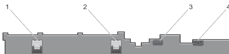
Figure 50. Vue arrière du fond de panier de huit disques durs
