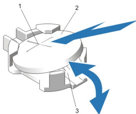
Figure 44. Remplacement de la pile du système
