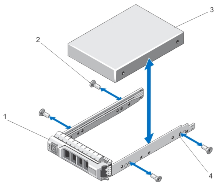
Figure 24. Retrait ou installation d'un disque dur remplaçable à chaud dans un support de disque dur
