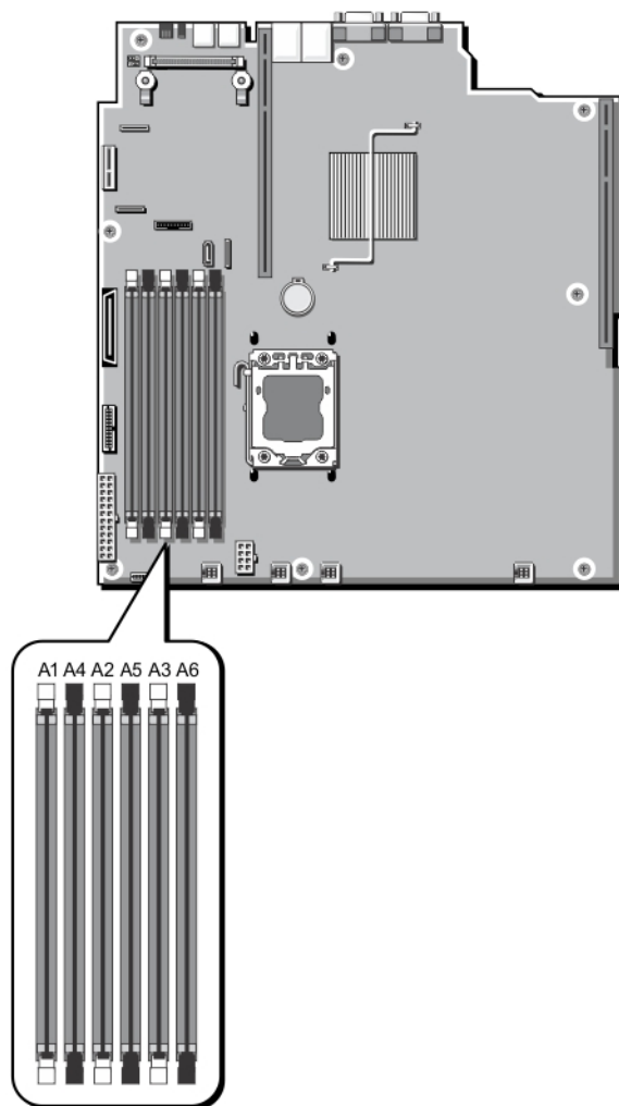
Figure 15. Emplacement des supports de mémoire
