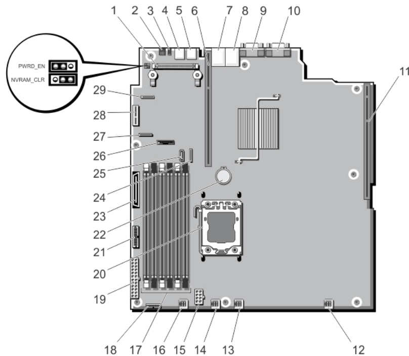
Figure 62. Connecteurs et cavaliers de la carte système
