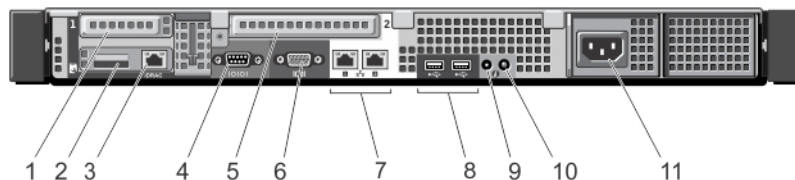
Figure 7. Voyants et fonctions du panneau arrière (avec bloc d'alimentation non-redondant)
