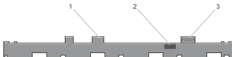
Figure 46. Vue arrière du fond de panier de quatre disques durs
