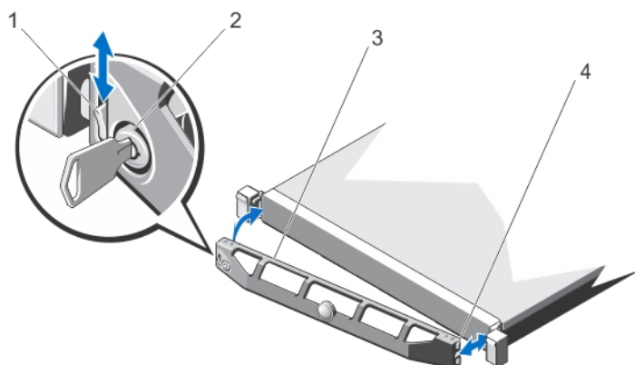
Figure 10. Installation et retrait du cadre avant
