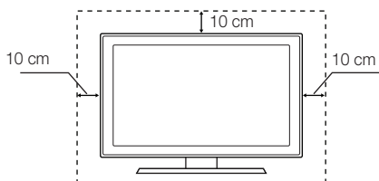
Montaż na podstawie
