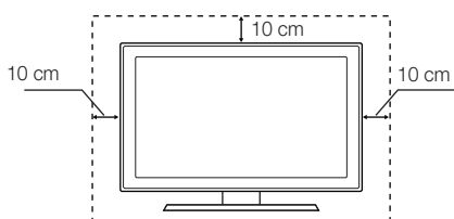
Montaža sa postoljem
