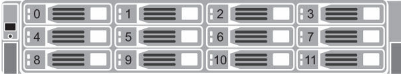
Figure 16. Numérotation des lecteurs d'Système de stockage SCv2000
