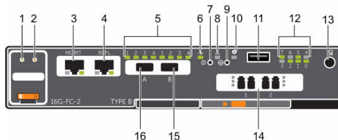
Figure 4. Contrôleur de stockage du Système de stockage SCv2000/SCv2020 avec deux ports avant Fibre Channel 16 Gb
