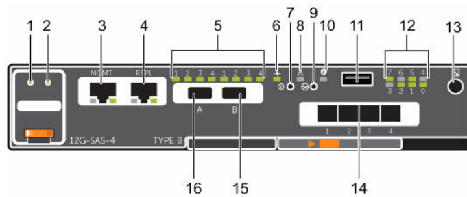
Figure 7. Contrôleur de stockage du Système de stockage SCv2000/SCv2020 avec quatre ports SAS avant 12 Gbits
