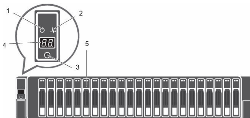
Figure 1. Vue du panneau avant du Système de stockage SCv2000/SCv2020
