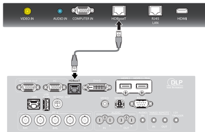
Projektoranschlüsse
