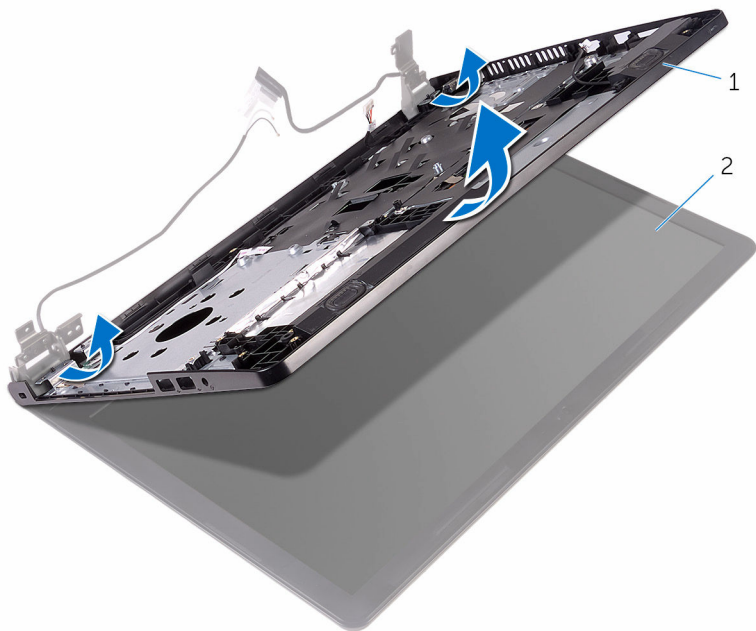
1 掌垫部件
