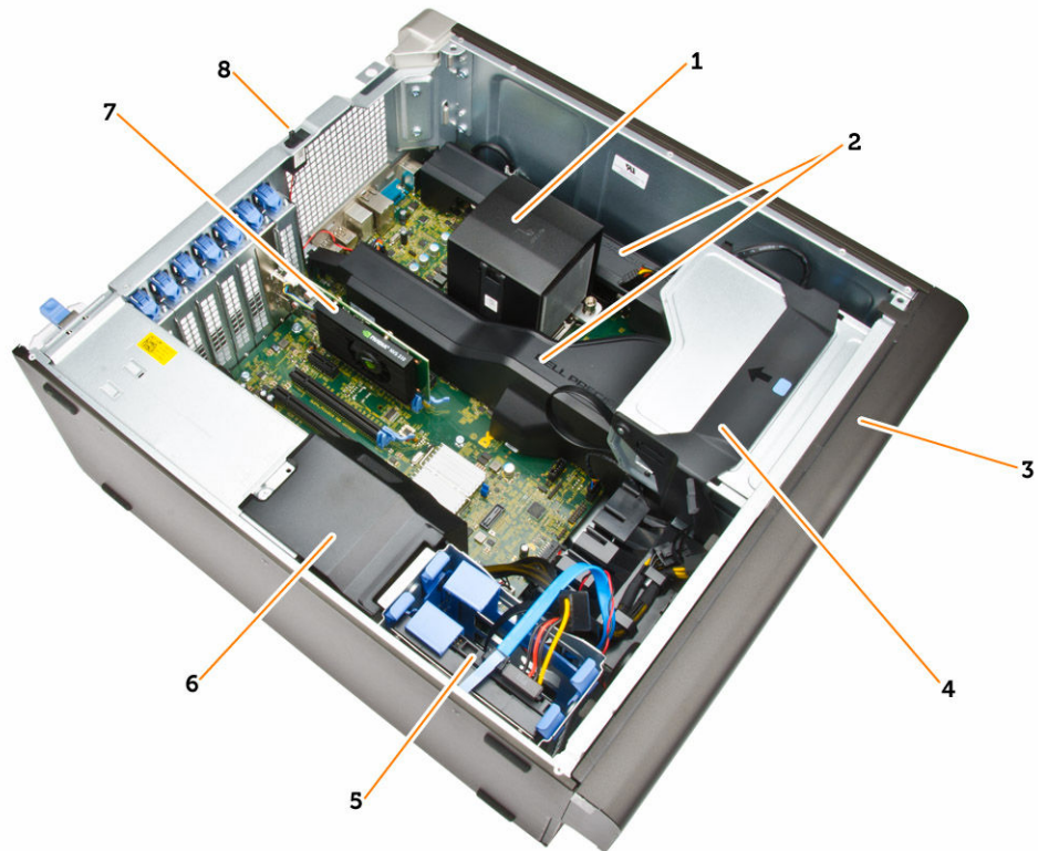
Afbeelding 2. Binnenaanzicht van de T5810 computer
