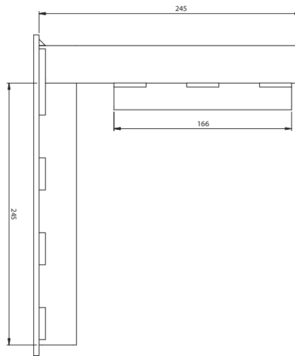
Seitenansicht
