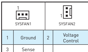
Connecteurs pour ventilateurs en mode tension
