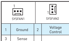
電圧モードファンコネクタ
