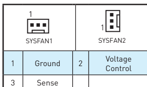
Разъем вентилятора с управлением постоянным током
