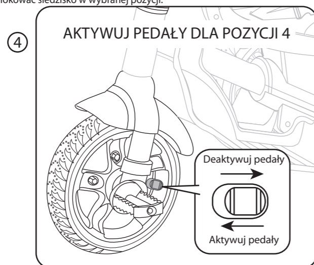
Wciśnij przycisk. Następnie go przesunij. Jeżeli nie udaje się przesunąć przycisku, obróć pedał.
