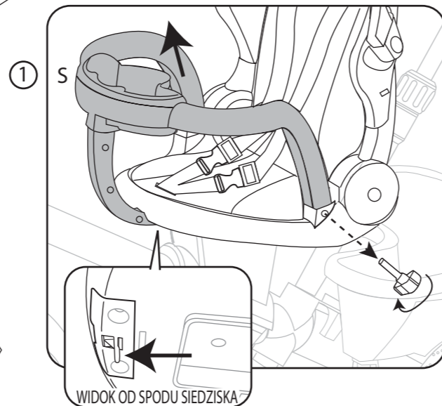
Zdemontuj barierkę zabezpieczającą (S): odkręć śruby po obu stronach barierki zabezpieczającej i unieś barierkę. Następnie dociskając w przód blokadę pod siedziskiem zwolnisz mocowanie barierki. Zdejmij barierkę.
