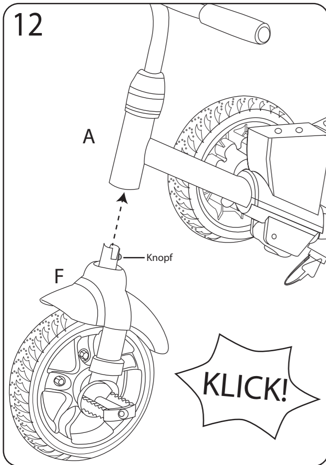
12 Rahmen (A) und Vorderrad (F) ineinander drücken und Knopf einrasten lassen.
