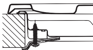
Position du crochet pour top H=40mm Derrière
