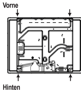
Position der Haken für Arbeitsplatten H=30mm
