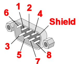
Pinbelegung des 9-Pin D-Sub Anschlusses
