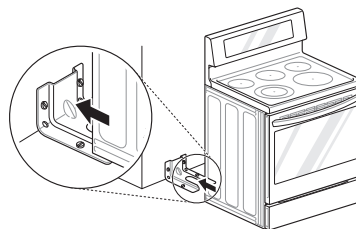
Enclencher le dispositif antibasculement
