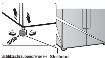
Schlitzschraubendreher (-) Stellhebel
