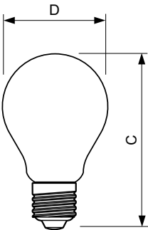
filament 7W-60W 620lm NAD 2200K E27D
