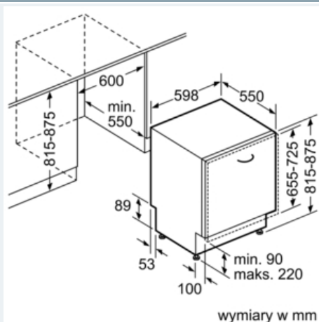
Rysunki wymiarowe
