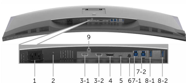
Widok od dołu monitora bez stojaka
