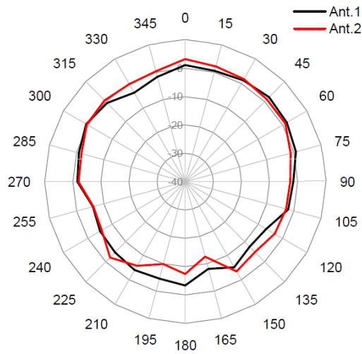
2.4GHz H-Plane
