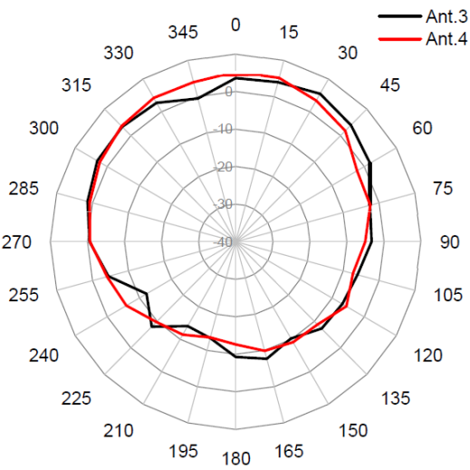
5GHz E-Plane
