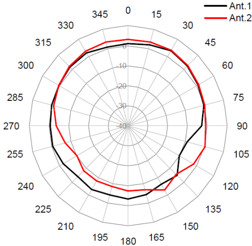
2.4GHz E-Plane
