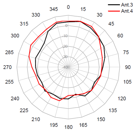
5GHz H-Plane
