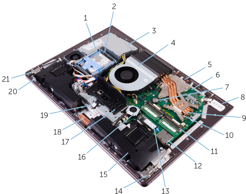
Abbildung 2. : Innenansicht des Computers (Non-Touchscreen)
