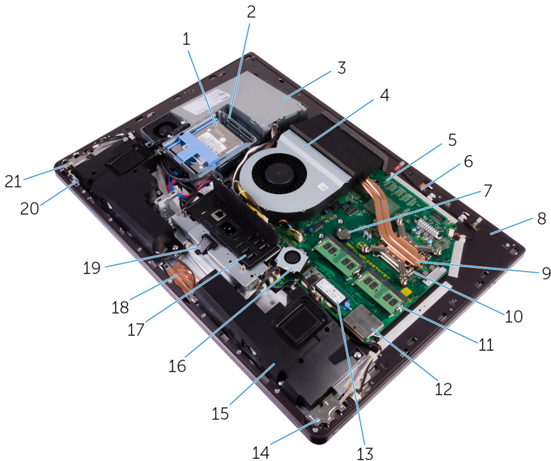
Abbildung 1. : Innenansicht des Computers
