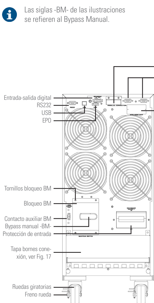
De 15 y 20 kVA B1. Entrada trifásica y salida monofásica.
