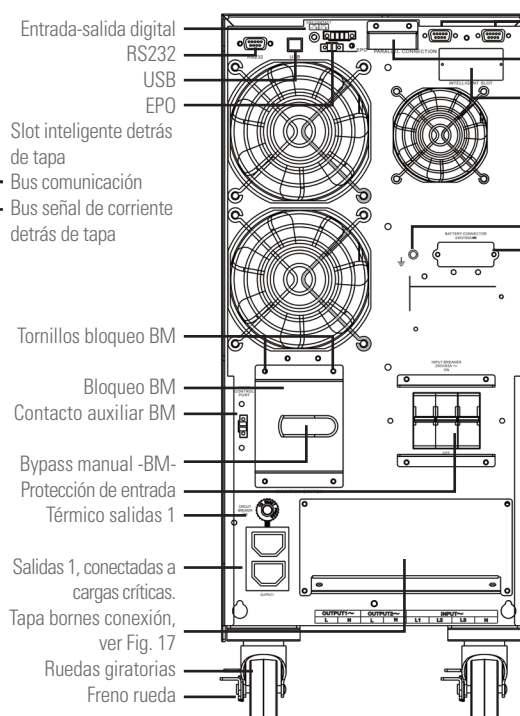
De 8 a 10 kVA estándar y B1. Entrada trifásica y salida monofásica.
