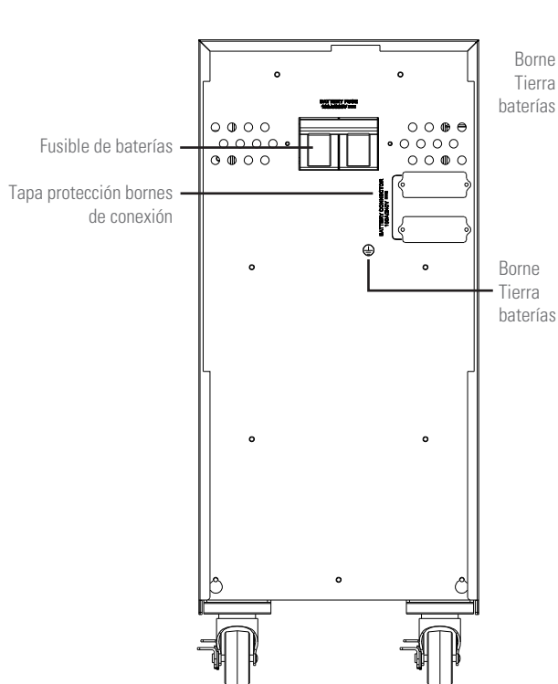
Módulo de baterías tamaño 1, con 2x20 elementos y protección de 100 A.
