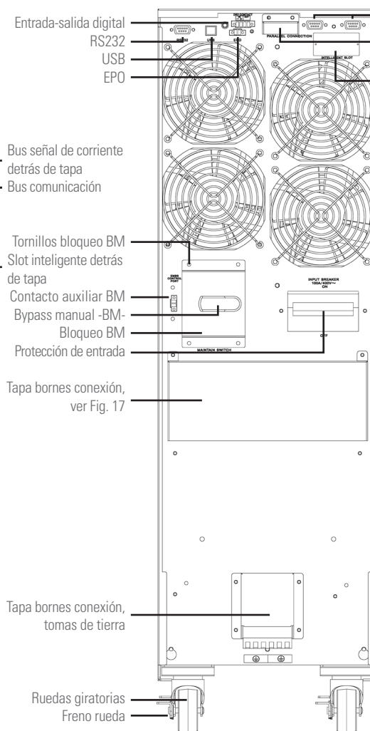
De 15 y 20 kVA estándar. Entrada trifásica y salida monofásica.
