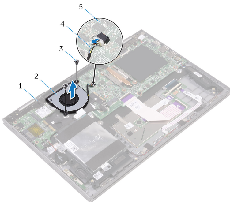
Figure 14. Fan
