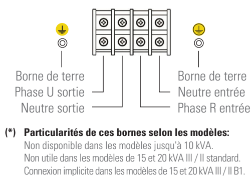
Réglette de bornes TWIN PRO2 4.. 10 kVA
