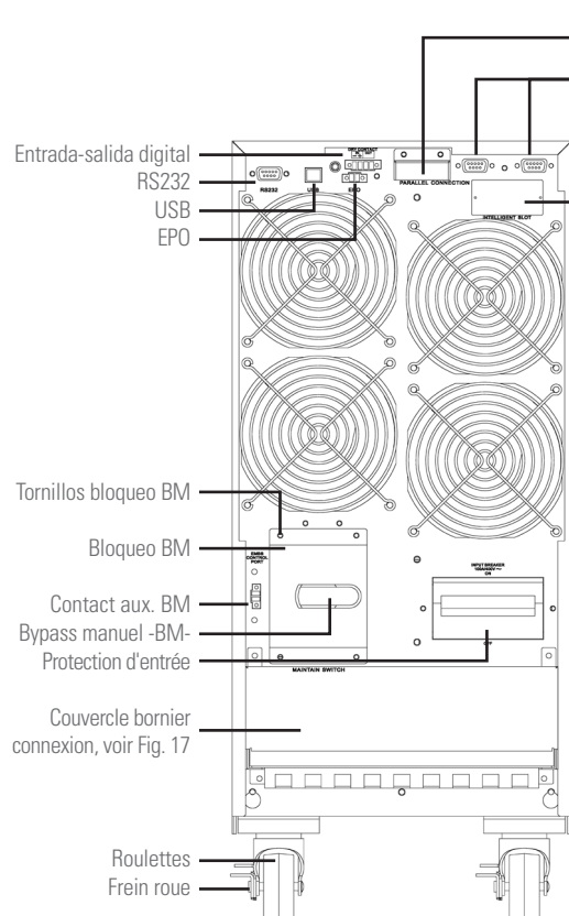
15 et 20 kVA B1. Entrée triphasée et sortie monophasée.
