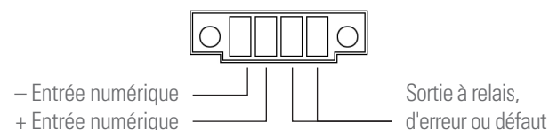
Fig. 20. Connecteur Entrée numérique-Sortie à relais.
