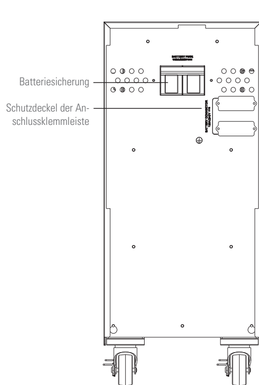
Batterieminodul GröÖe 1, mit 2x20 Elementen und Schutz von 100 A.
