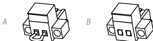
Abb. 19. Stecker für den externen Not-Aus-Schalter.
