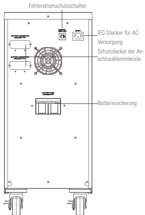
Batterieminodul GröÖe 1, mit 3x20 Elementen und Schutz von 100 A.
