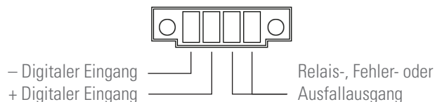
Abb. 20. Digitaler Eingangsstecker und Ausgangsrelais.
