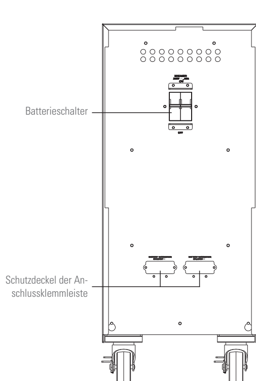
Batterieminodul GröÖe 1, mit 2x20 Elementen und Schutz von 50 A.
