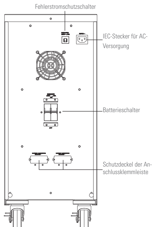
Batterieminodul GröÖe 1, mit 3x20 Elementen und Schutz von 50 A.
