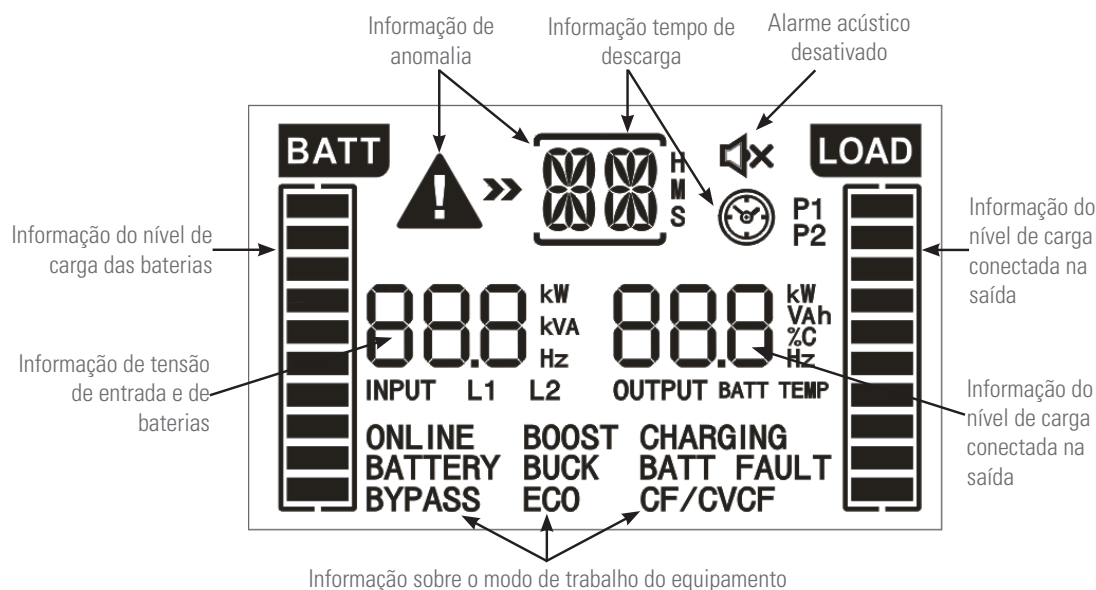
Fig. 27. Painel de controlo com monitor LCD.
