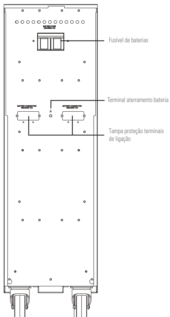
Módulo de baterias tamanho 2, com 4x20 elementos e proteção de 100 A.
