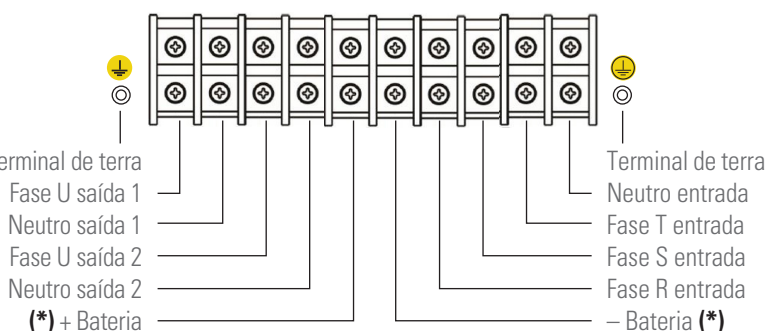
Barra de terminais TWIN/3 PRO2 8.. 20 kVA
