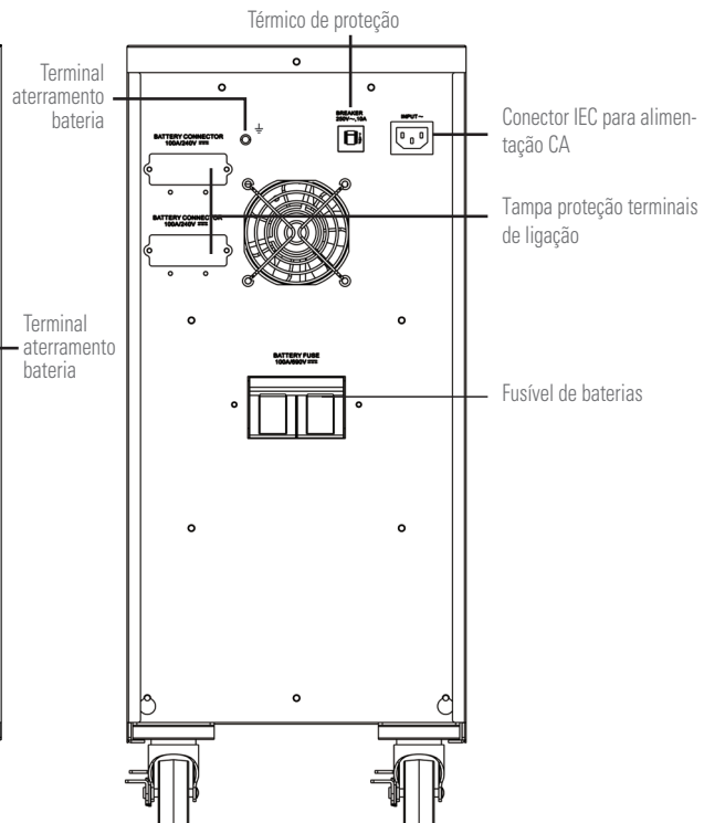
Módulo de baterias tamanho 1, com 3x20 elementos e proteção de 100 A.
