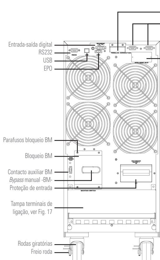
Fig. 2. Vista posterior modelos de 4 kVA a 20 kVA.
