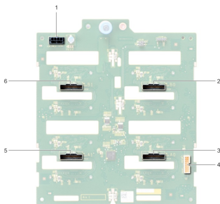
Ilustración 95. Backplane de unidad NVMe de 8 x 2,5 pulgadas
