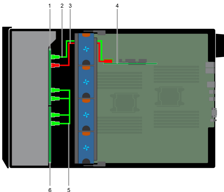
Ilustración 100. SAS/SATA x32 de 2,5 pulgadas a PERC interna
