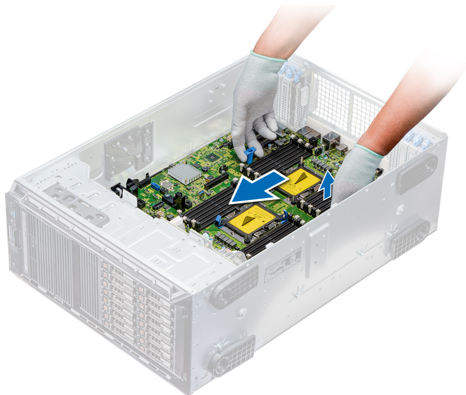
Ilustración 118. Desbloqueo de la tarjeta madre del sistema
