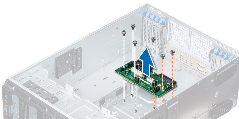
Ilustración 125. Extracción de la PIB principal
