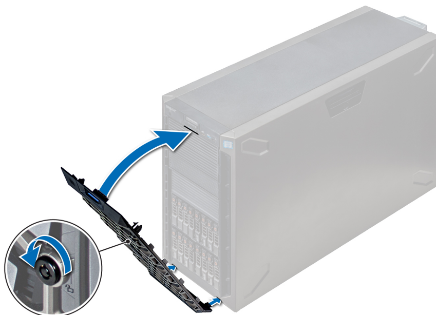
Ilustración 21. Instalación del bisel frontal
