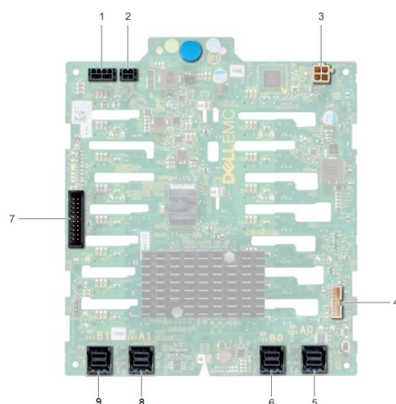
Ilustración 93. Backplane SAS o SATA de 16 x 2,5 pulgadas para FlexBay (superior)
