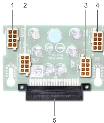
Ilustración 122. Tarjeta mediadora de alimentación de GPU
