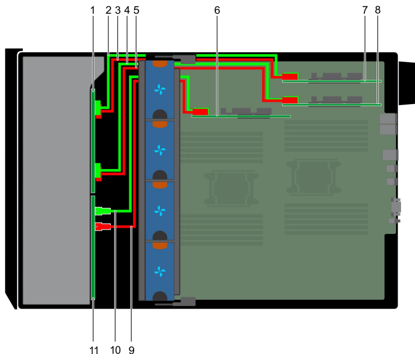
Ilustración 102. SAS/SATA x16 de 2,5 pulgadas a PERC interna con NVMe x8 de 2,5 pulgadas a puente PCIe
