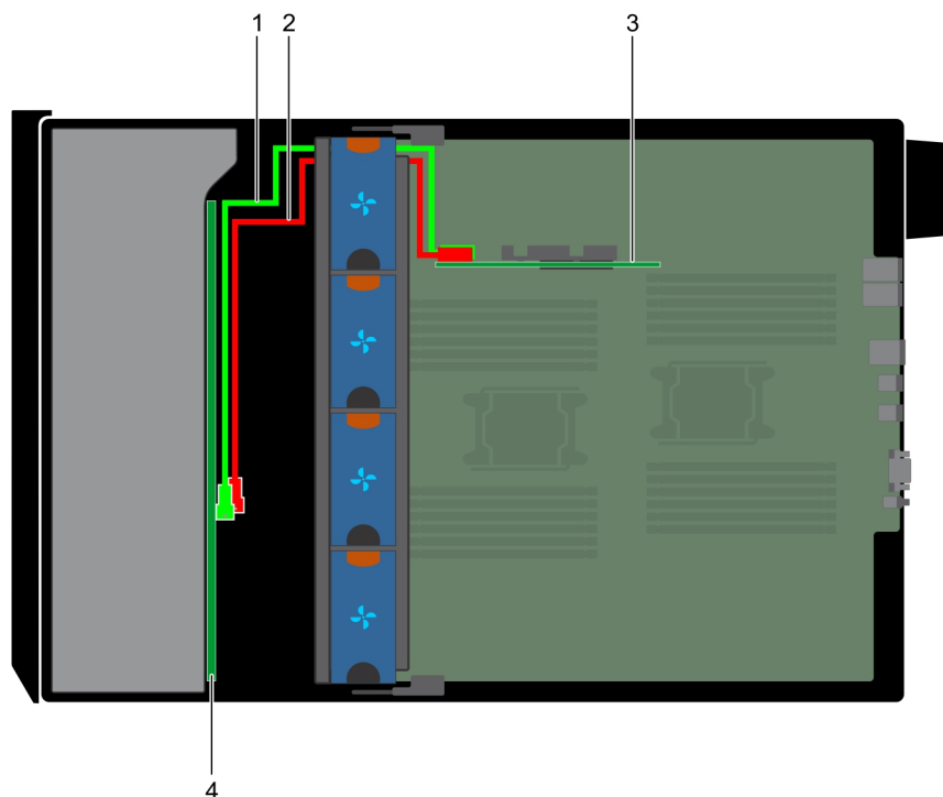
Ilustración 107. PERC interna x18 de 3,5 pulgadas
