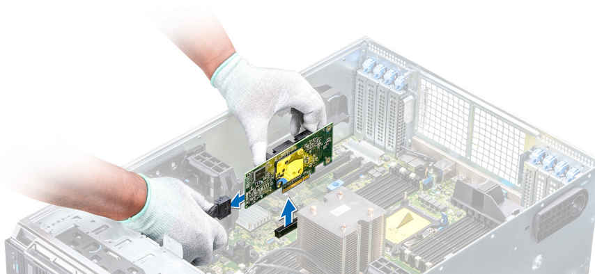
Ilustración 109. Extracción de la tarjeta controladora de almacenamiento integrada
