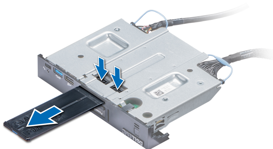
Ilustración 114. Extracción de la etiqueta de información
