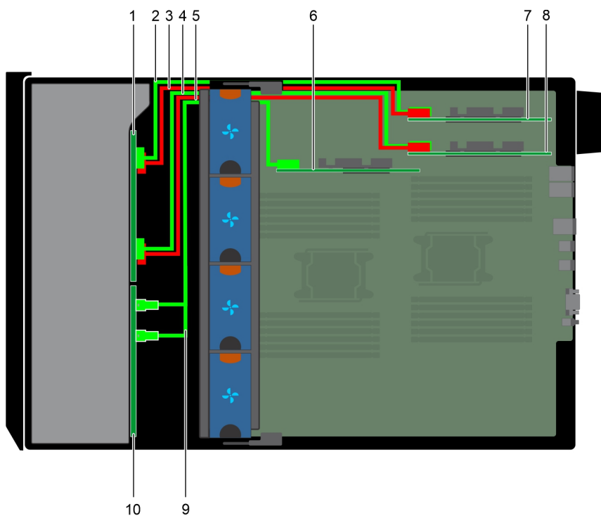
Ilustración 103. SAS/SATA x16 de 2,5 pulgadas a PERC interna con NVMe x8 de 2,5 pulgadas a puente PCIe
