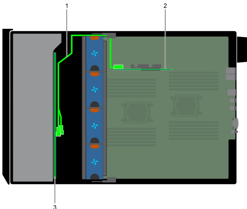
Ilustración 108. PERC interna x18 de 3,5 pulgadas
