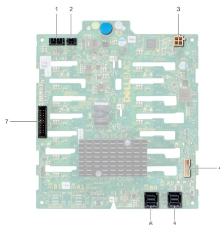
Ilustración 94. Backplane SAS o SATA de 16 x 2,5 pulgadas
