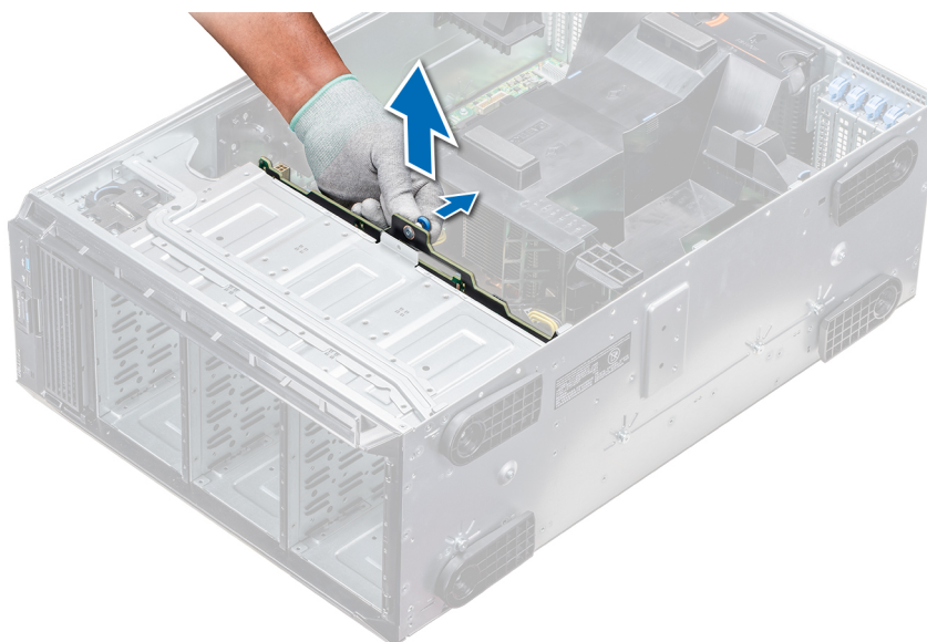
Ilustración 98. Extracción de un backplane
