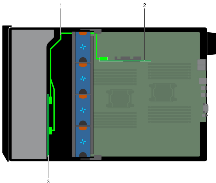
Ilustración 105. SAS/SATA x8 de 3,5 pulgadas a PERC interna
