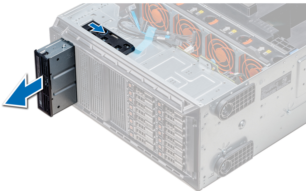
Ilustración 56. Extracción de la caja de la unidad óptica o la unidad de cinta
