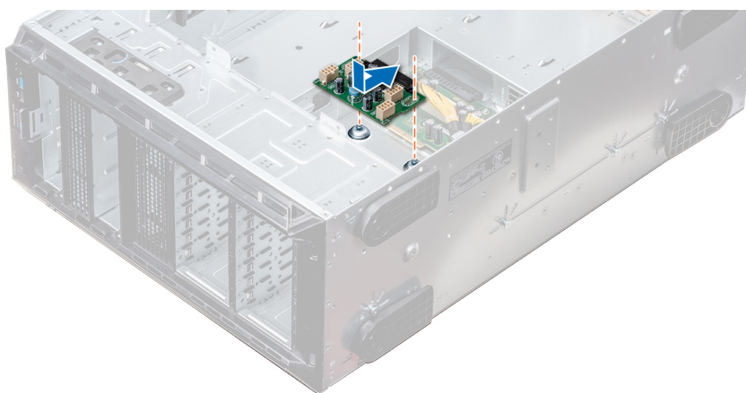
Ilustración 124. Instalación de la tarjeta mediadora de alimentación de GPU
