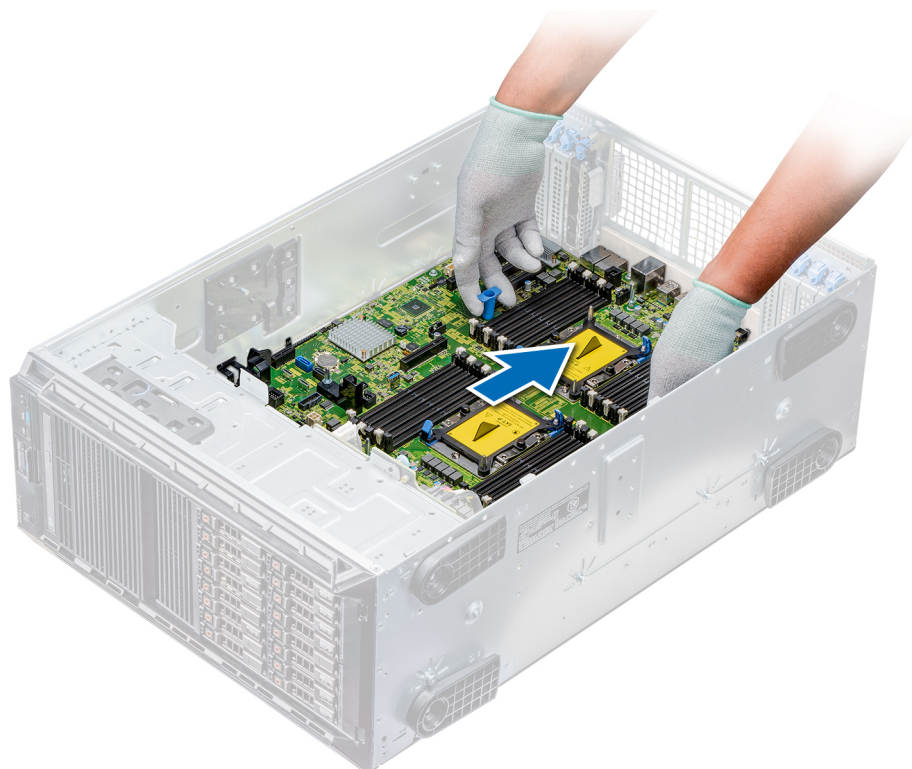
Ilustración 120. Instalación de la tarjeta madre
