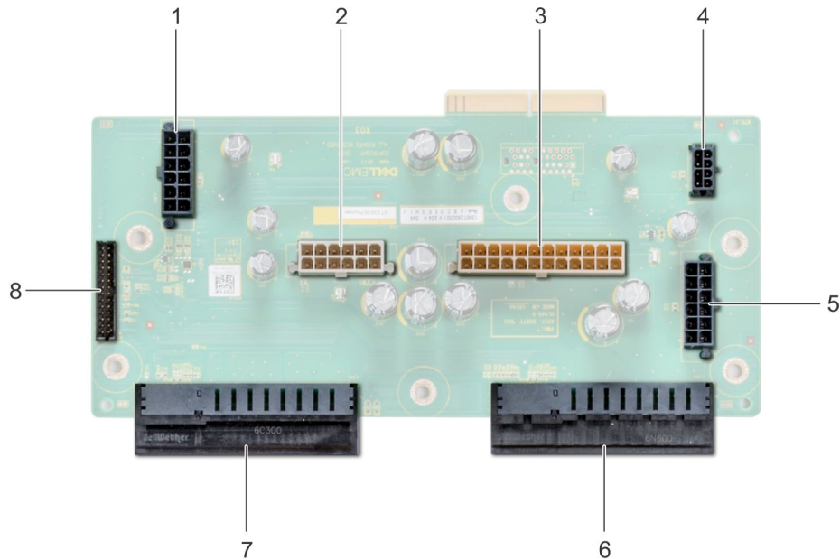
Ilustración 121. Tarjeta mediadora de alimentación principal
