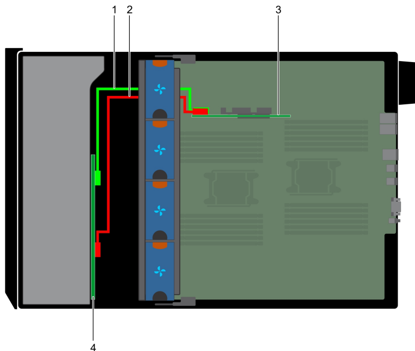
Ilustración 104. SAS/SATA x8 de 3,5 pulgadas a PERC interna
