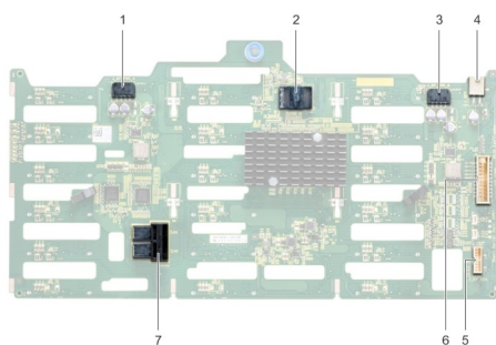
Ilustración 96. Backplane SAS o SATA de 18 x 3,5 pulgadas
