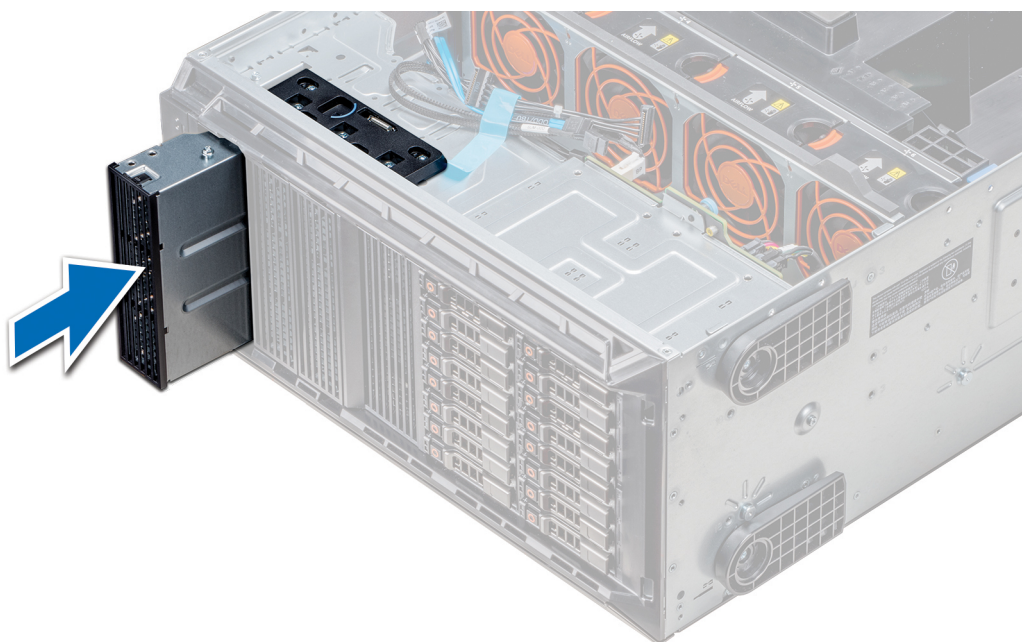
Ilustración 55. Instalación de la unidad óptica o de cinta de relleno
