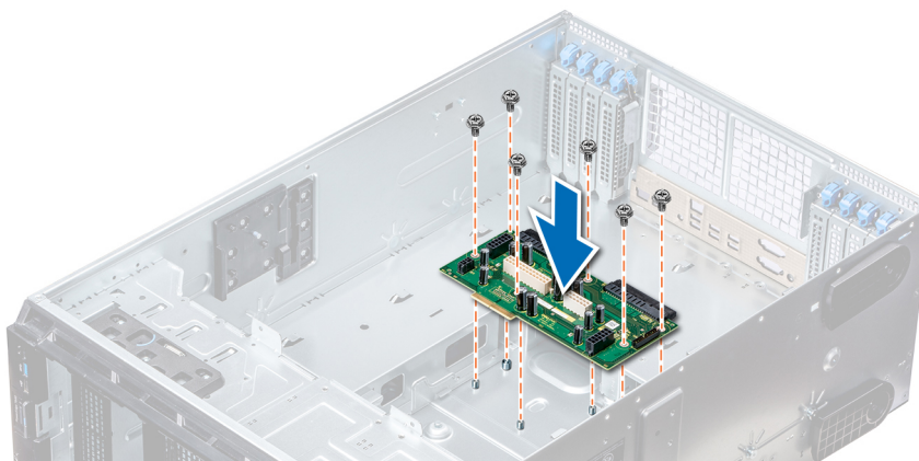
Ilustración 126. Instalación de la placa mediadora de alimentación principal
