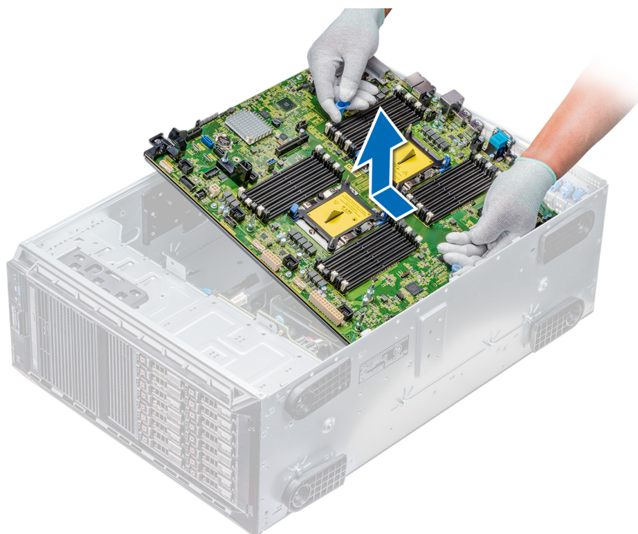
Ilustración 119. Extracción de la placa base
