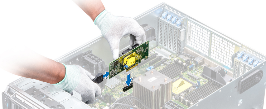
Ilustración 110. Instalación de la tarjeta controladora de almacenamiento integrada
