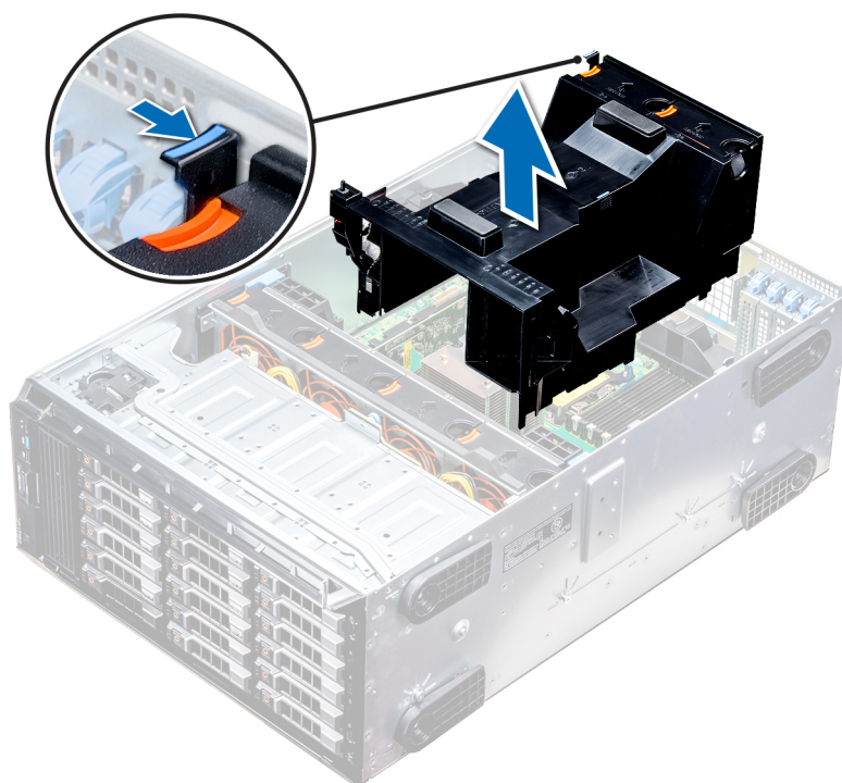
Ilustración 44. Extracción de la cubierta para flujo de aire
