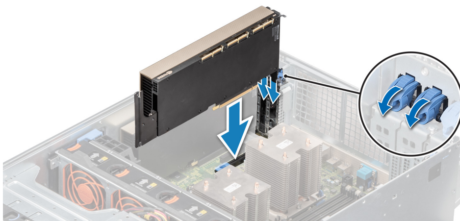
Ilustración 83. Instalación de la tarjeta de GPU opcional
