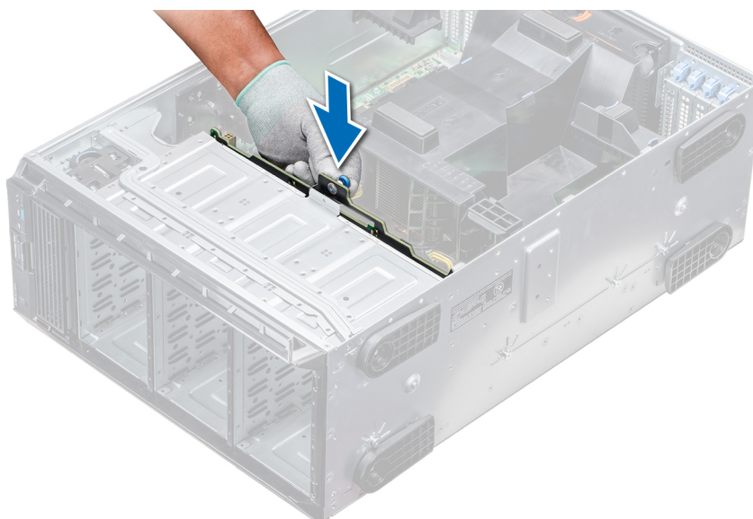
Ilustración 99. Instalación de un backplane
