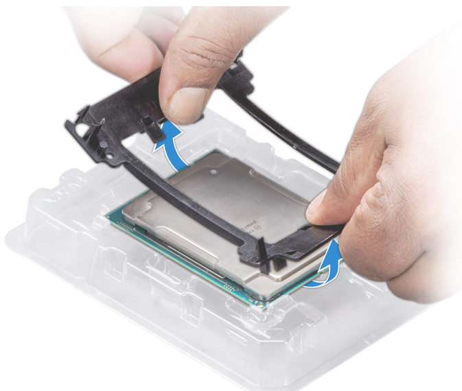
Ilustración 67. Extracción del soporte del procesador
