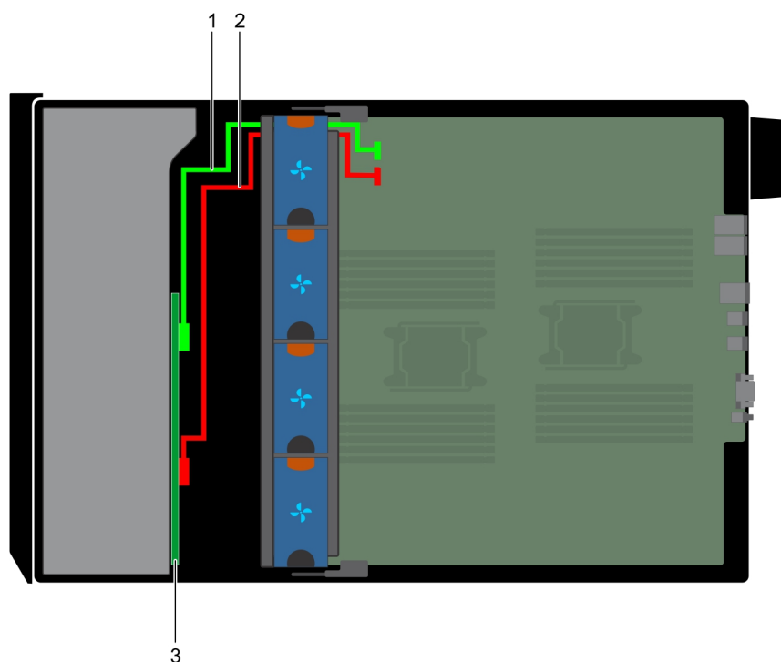
Ilustración 106. Controladora SAS a bordo x8 de 3,5 pulgadas
