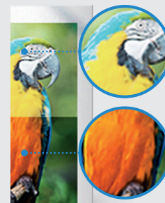
Verschwommene Bilder
