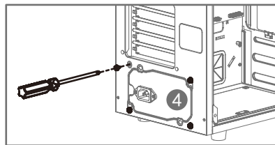
电源安装：拆掉④
