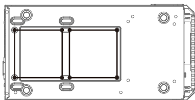
机箱底部：支持120mmX2风扇
