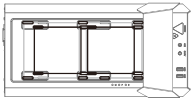
机箱顶部： 支持120mmX2或140mmX2风扇或120/140/240mm水冷排
