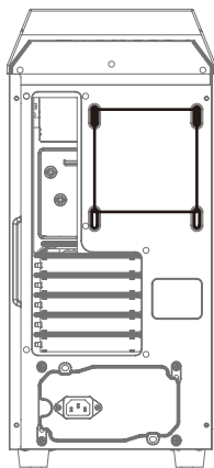
机箱后部： 支持120mm风扇或120mm水冷排
