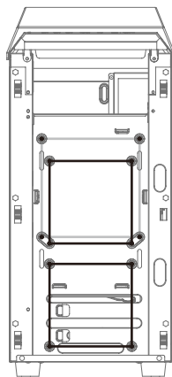
机箱前部： 支持120mmX2或120mm+140mm风扇
