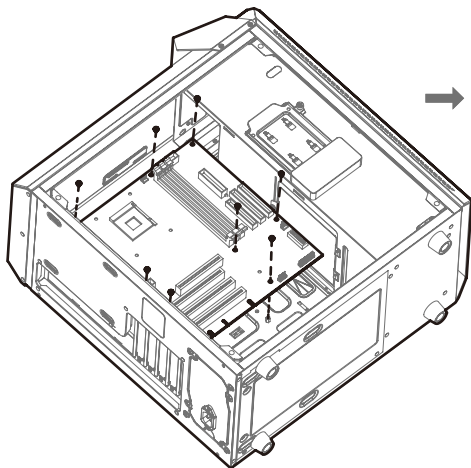
Mini-ITX、M-ATX主板安装
