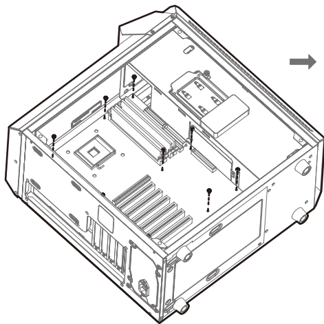
ATX主板安装
