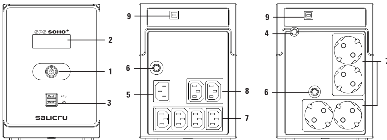
Abb. 2. Ansicht der Modelle SPS.SOHO+ 1200/1600 VA.
