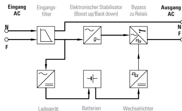
Abb. 4. Strukturelles Blockschema.
