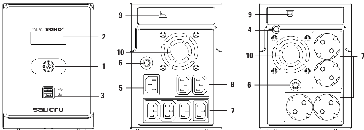
Abb. 3. Ansicht der Modelle SPS.SOHO+ 2200 VA.
