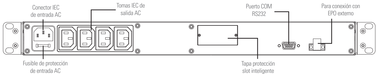
Fig. 2. Vista posterior SPS ADVANCE R.
