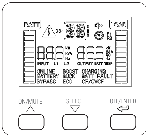
Fig. 14. Vue du panneau de commande.
