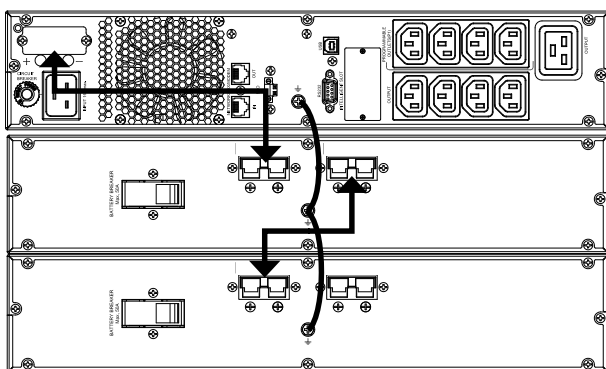
Fig. 9. Connexion avec modules de batteries.
