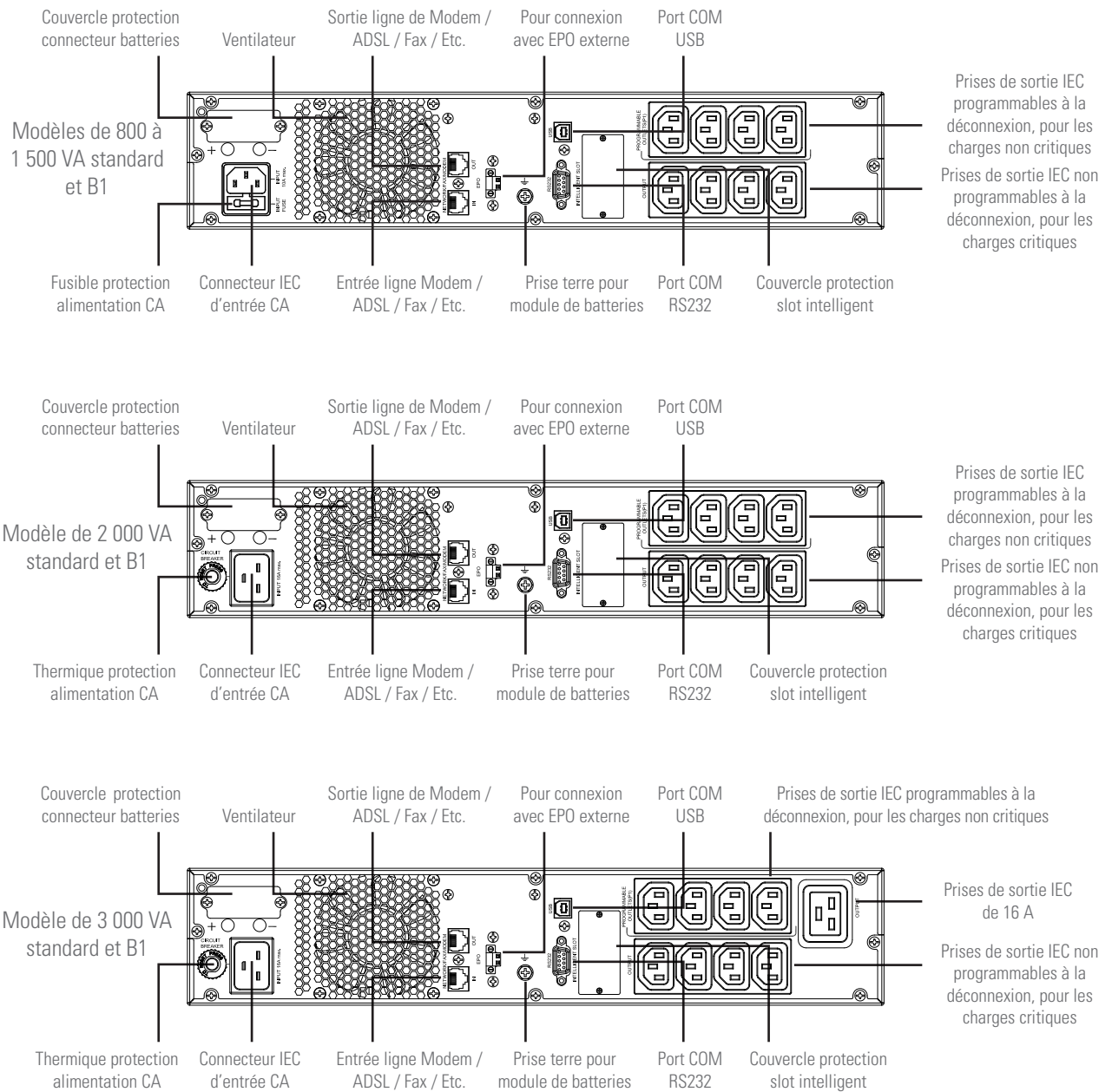
Fig. 2. Vues arrière en fonction de la puissance des équipements.
