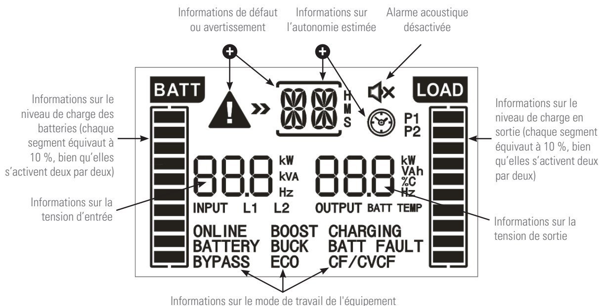
Fig. 13. Informations graphiques et textuelles affichées à l'écran.
