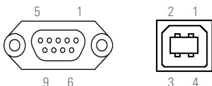
Fig. 11. Connecteurs DB9 pour RS232 et USB.
