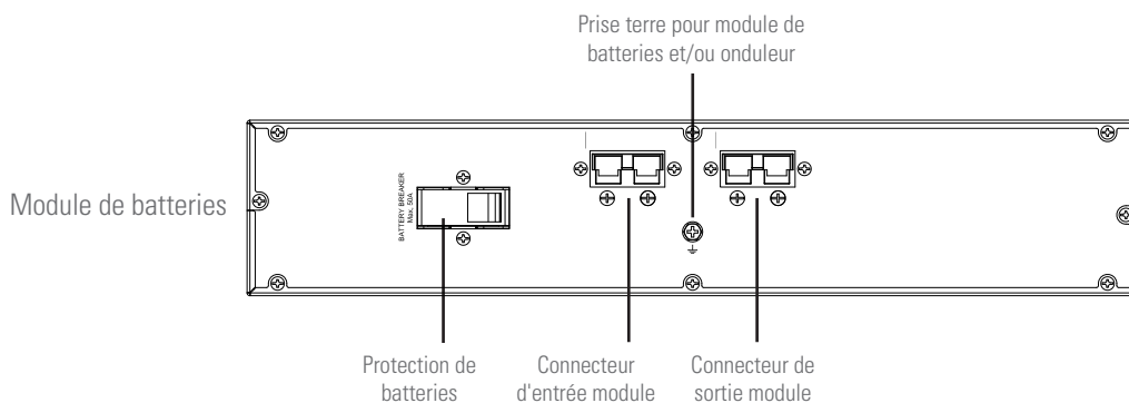
Fig. 2. Vues arrière en fonction de la puissance des équipements.
