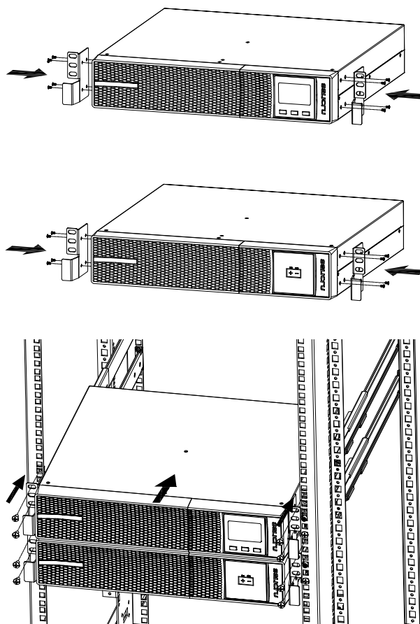
Fig. 5. Montage type rack en armoire de 19", avec extension autonomie (module de batteries).
