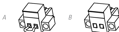
Fig. 10. Connecteur pour l'EPO externe.
