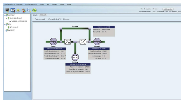
Fig. 12. Vue écran principal logiciel de surveillance ViewPower.
