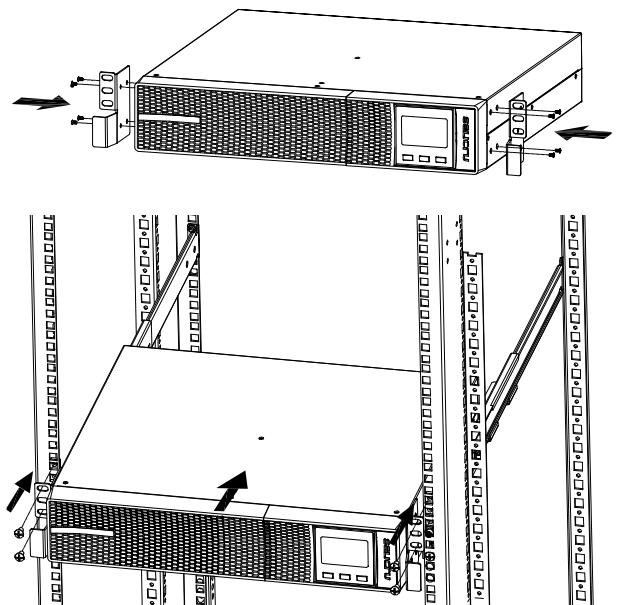
Abb. 4. Montage Typ Rack im 19"-Schränk.
