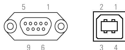
Abb. 11. Stecker DB9 für RS232 und USB.
