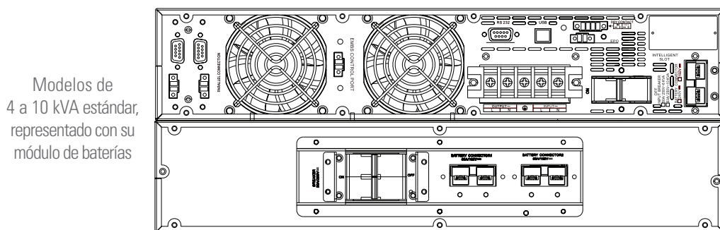
Fig. 2. Vista posterior modelos de 4 a 10 kVA.
