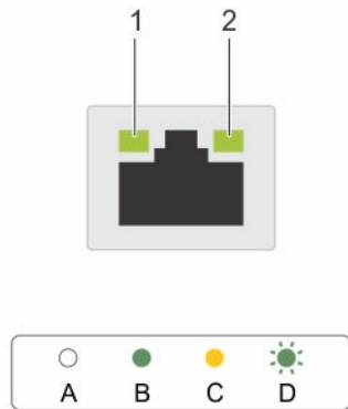
Abbildung 3. NIC-Anzeigen
