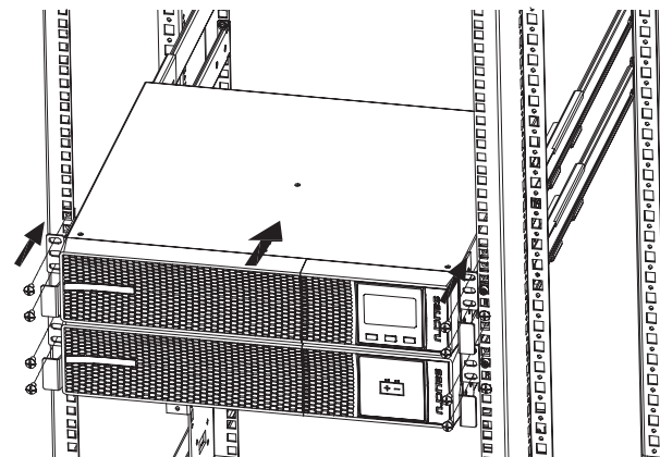
Fig. 9. Modelo en montaje rack en armario 19", con extensión autonomía (módulo de baterías).
