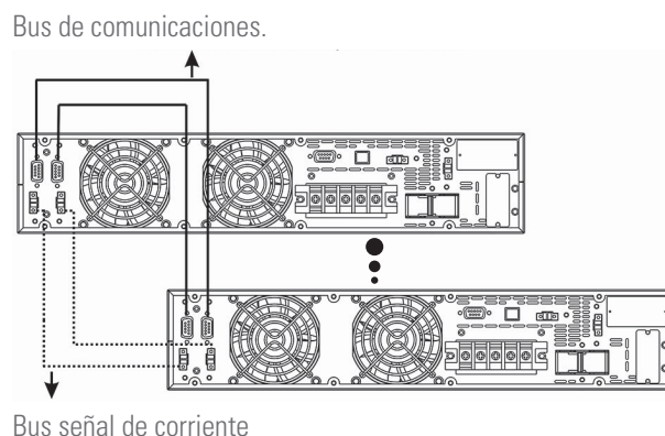
Fig. 17. Conexiones de comunicación y señal de corriente para sistema en paralelo.
