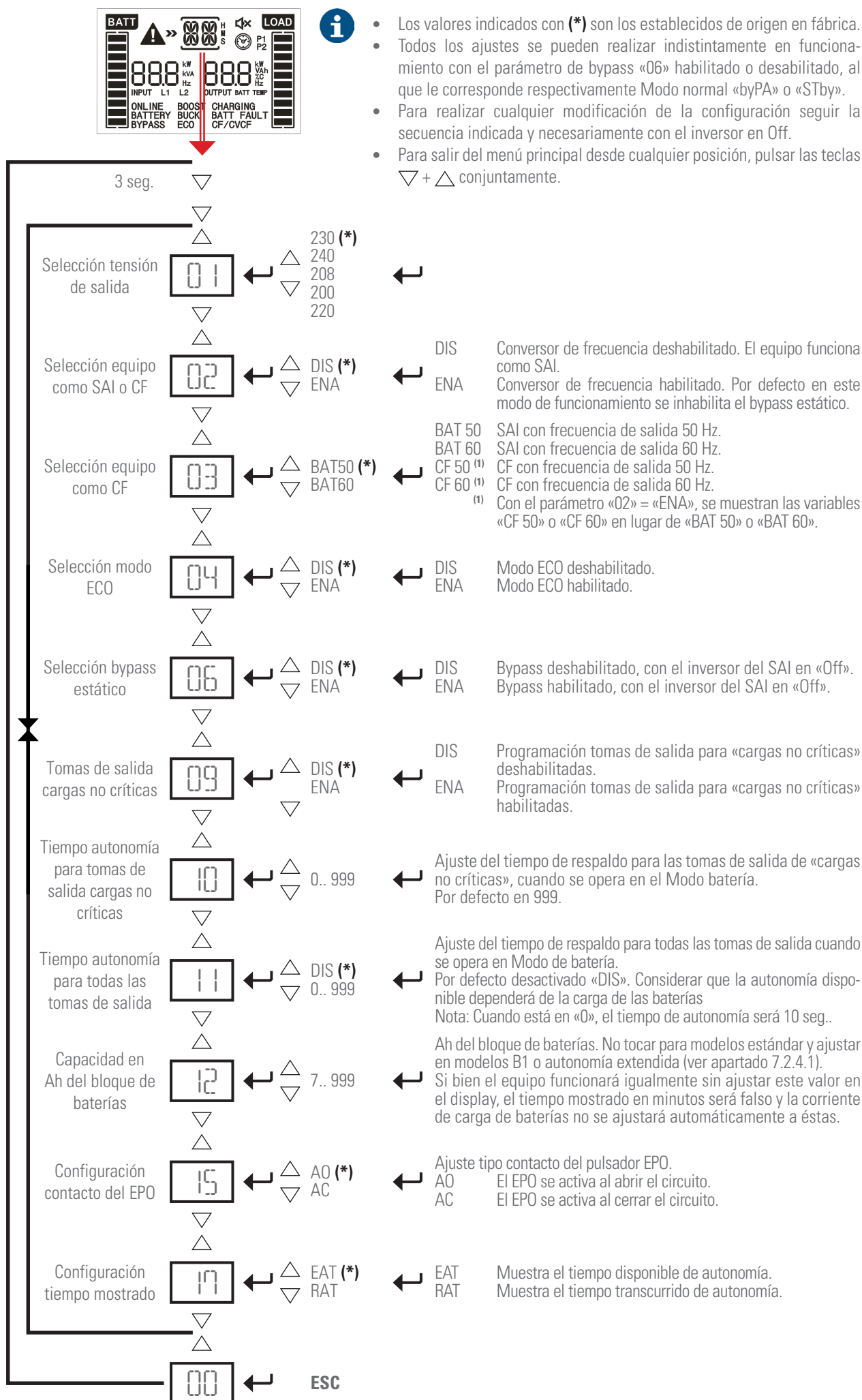
Fig. 24. Menú de ajustes.
