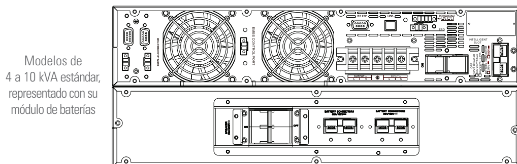
Fig. 2. Vista posterior modelos de 4 a 10 kVA.
