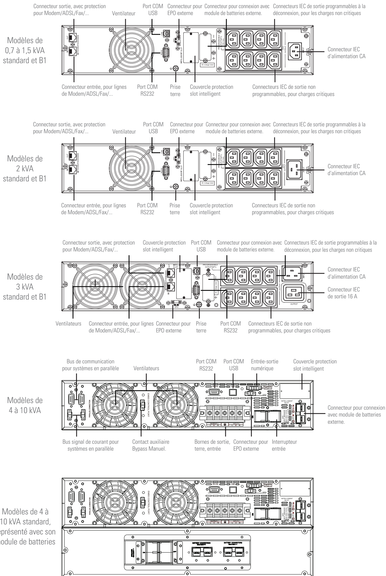
Fig. 2. Vue arrière modèles de 4 à 10 kVA.
