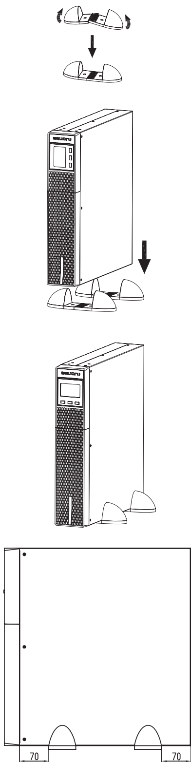
Fig. 6. Montagem vertical (tipo torre).
