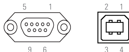
Fig. 19. Connecteurs DB9 pour RS232 et USB.
