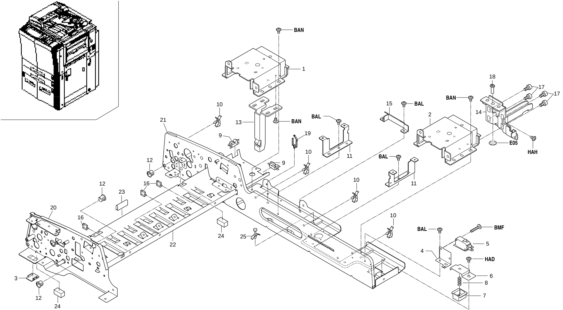
FIG. 32 FRAME SECTION (DF)
