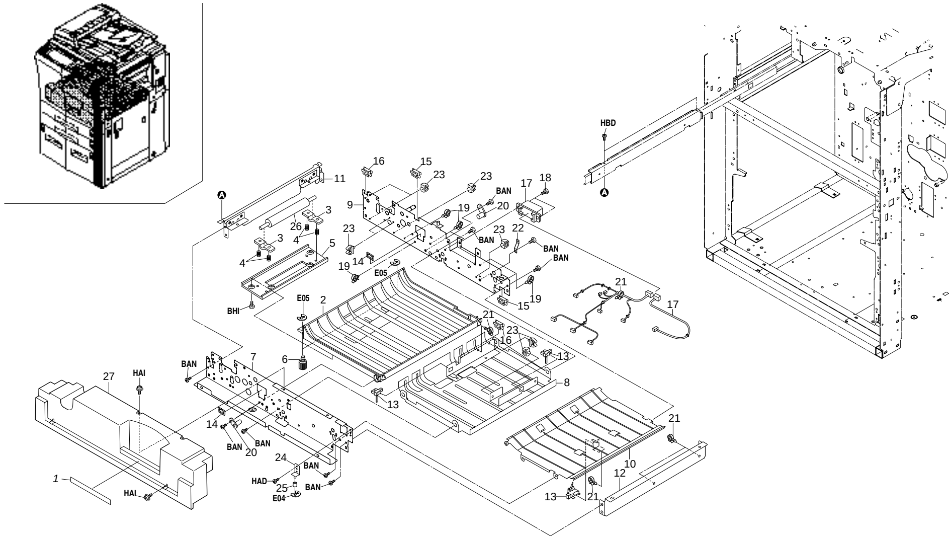
FIG. 23 DUPLEX SECTION I
