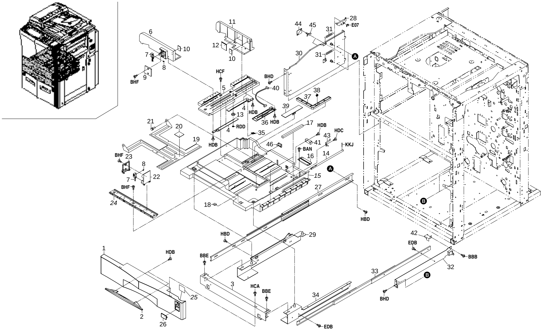
FIG. 3 CASSETTE SECTION
