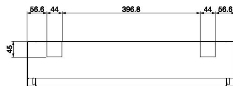
SEZIONE B-B
