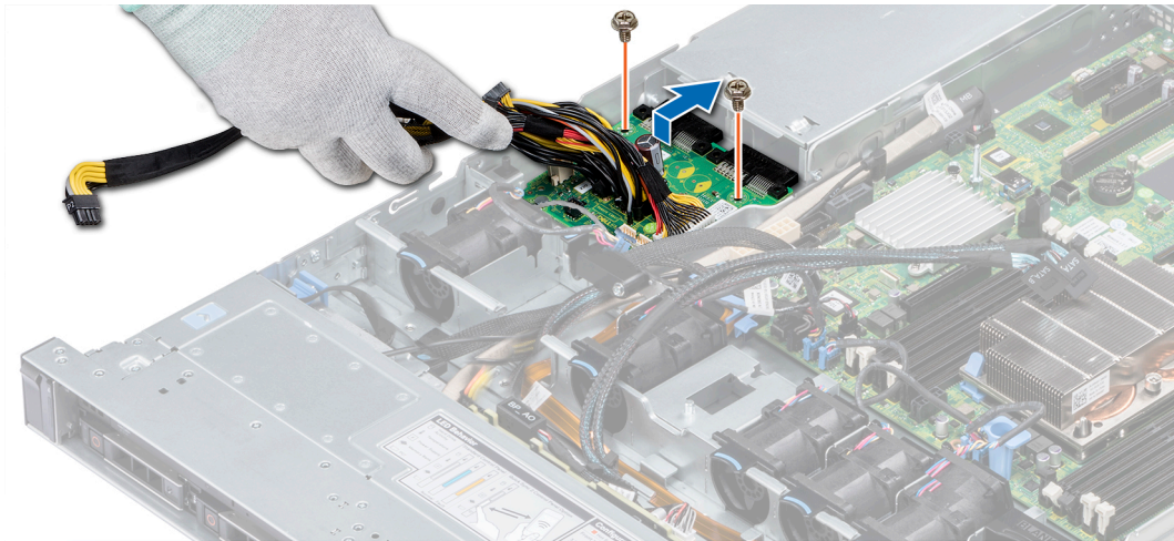
Abbildung 101. Entfernen der Stromzwischenplatine
