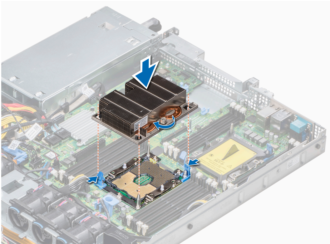
Abbildung 44. Installieren des Prozessor- und Kühlkörpermoduls
