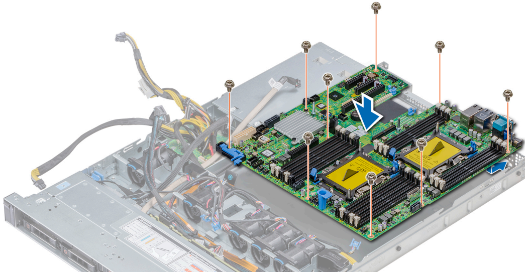
Abbildung 110. Einsetzen der Systemplatte
