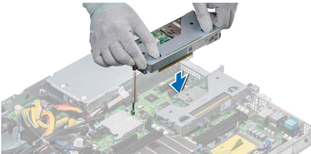
Abbildung 57. Installieren des Erweiterungskarten-Risers 2
