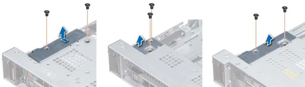
Abbildung 103. Entfernen der Kabelabdeckung
