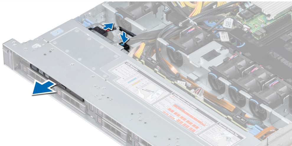
Abbildung 93. Entfernen des optischen Laufwerks
