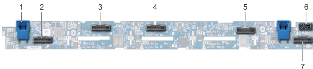
Abbildung 83. 10 x 2,5-Zoll-Rückwandplatine
