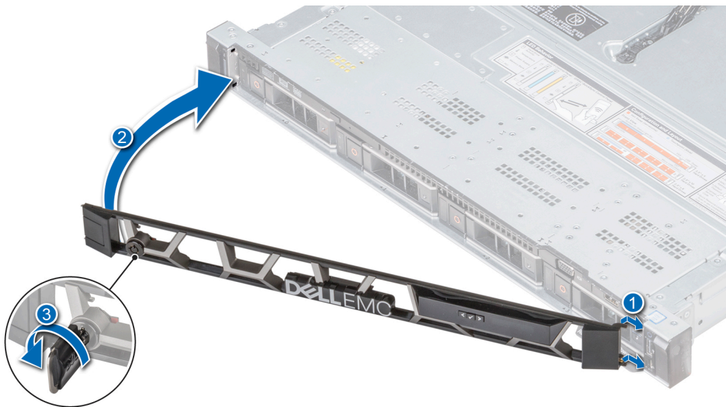
Abbildung 18. Anbringen der Frontblende mit LCD-Display
