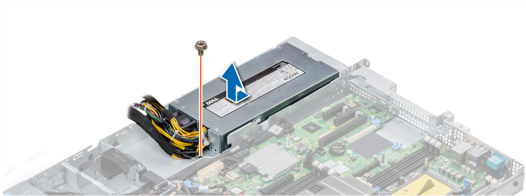
Abbildung 99. Entfernen eines nichtredundanten verkabelten Wechselstromnetzteils
