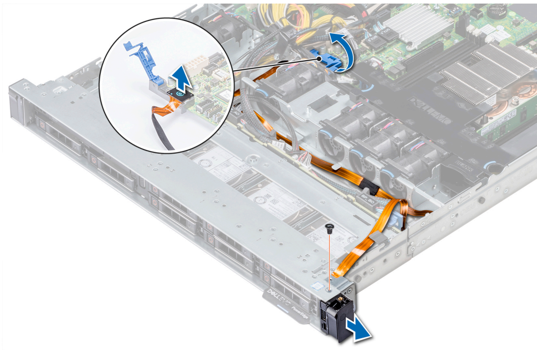
Abbildung 107. Entfernen des Bedienfelds
