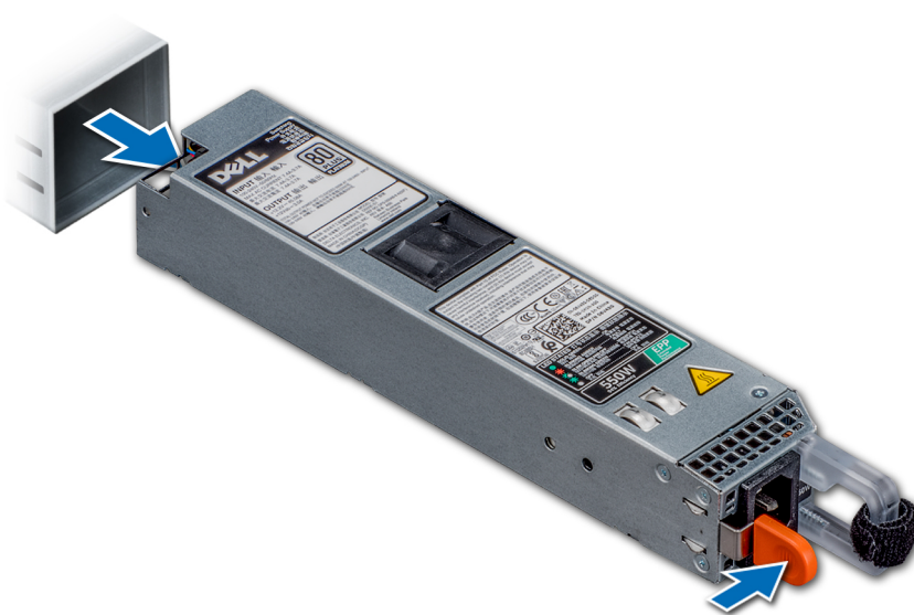
Abbildung 97. Entfernen eines Netzteils
