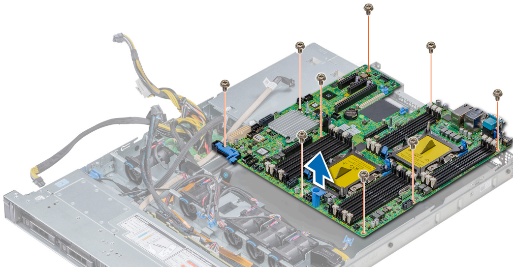
Abbildung 109. Entfernen der Systemplatine
