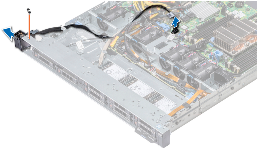
Abbildung 104. Entfernen des linken Bedienfelds
