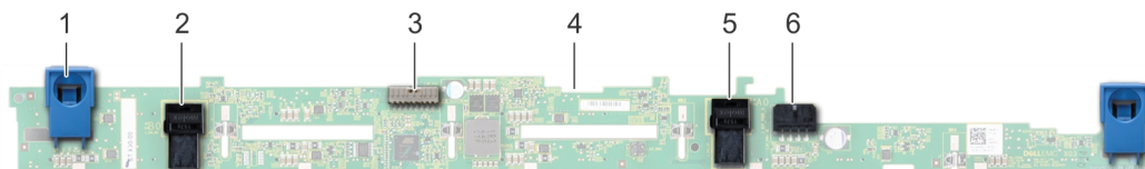
Abbildung 82. 8 x 2,5-Zoll-Rückwandplatine
