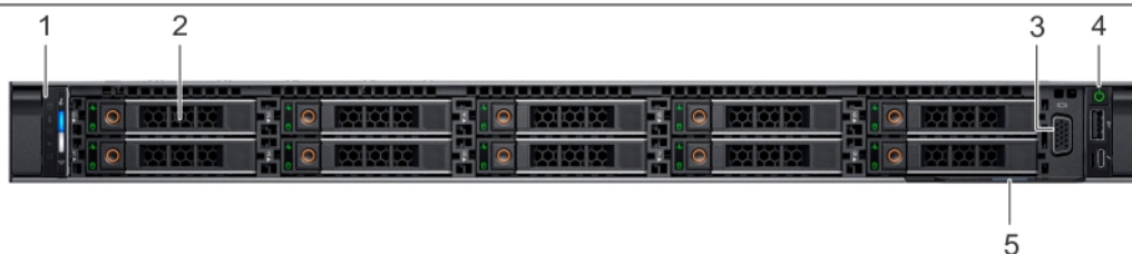
Abbildung 3. Frontansicht eines Systems mit 10 x 2,5-Zoll-Laufwerken
