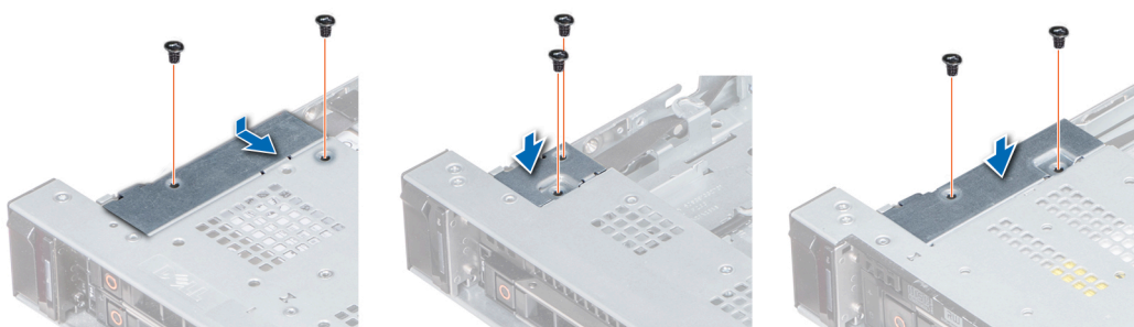
Abbildung 105. Installieren der Kabelabdeckung
