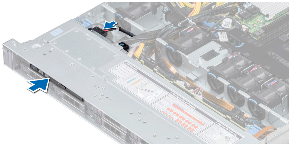
Abbildung 94. Installieren eines optischen Laufwerks
