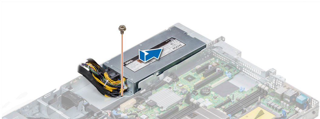
Abbildung 100. Installieren eines nichtredundanten verkabelten Wechselstromnetzteils
