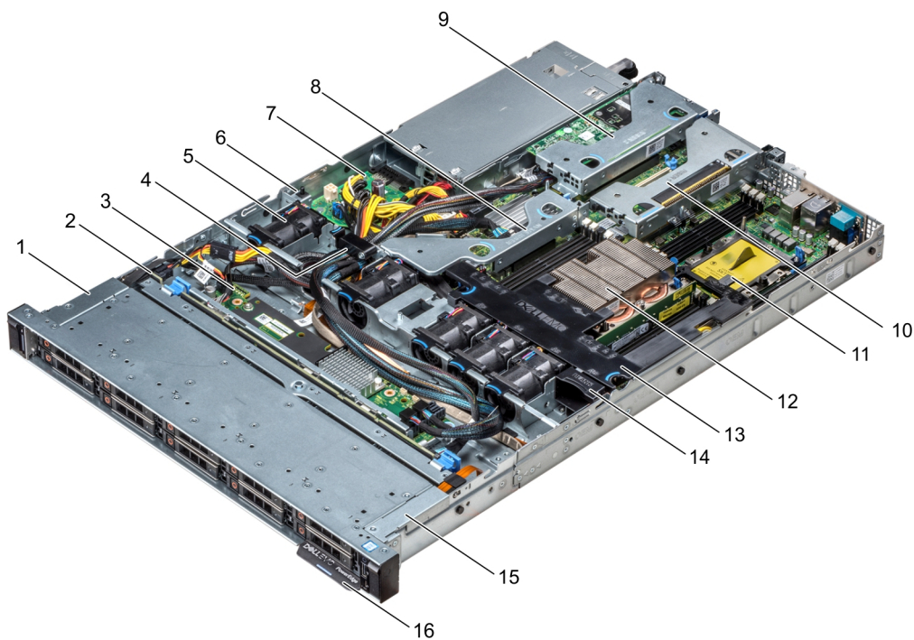
Abbildung 21. Das Systeminnere
