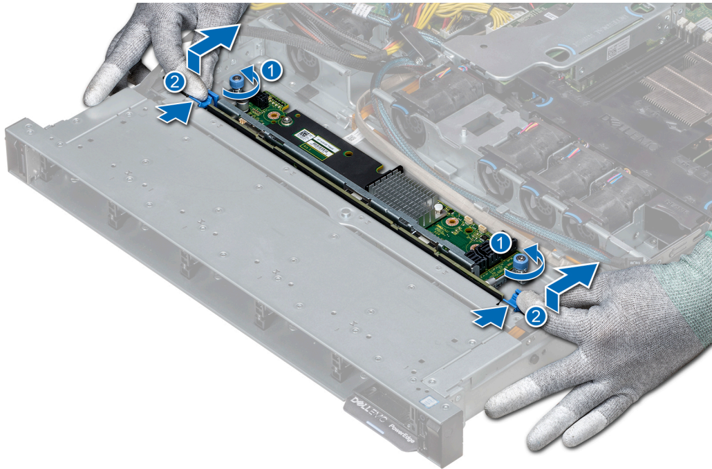
Abbildung 86. Entfernen der Festplatten-Rückwandplatine
