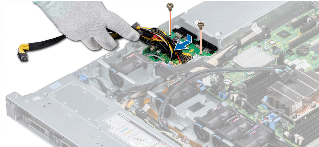
Abbildung 102. Installieren der Stromzwischenplatine
