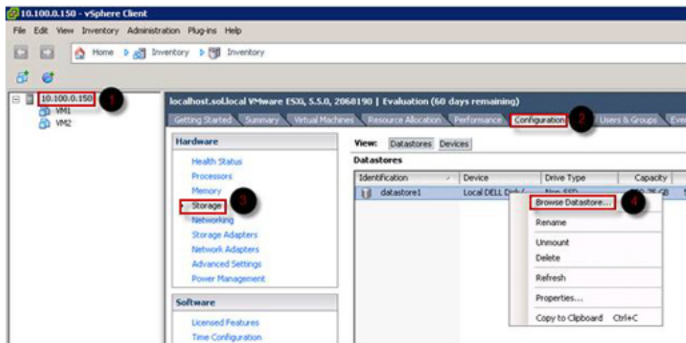
Abbildung 16. vSphere Client
