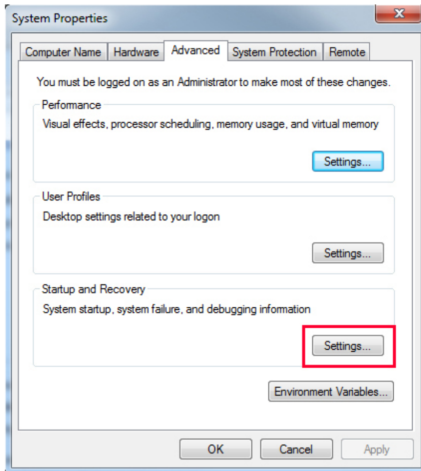
Abbildung 11. Fenster „Systemeigenschaften“
